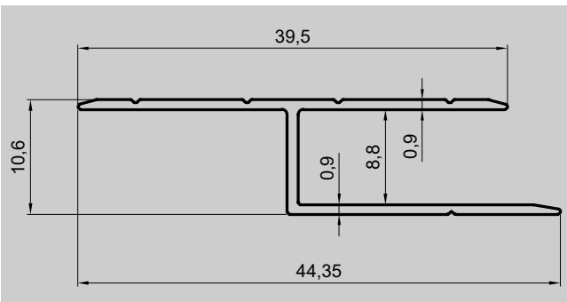
Teknik Çizim / Technical Drawing
