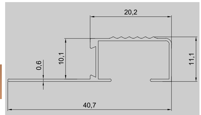
Teknik Çizim / Technical Drawing
