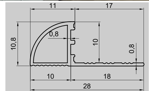
Teknik Çizim / Technical Drawing
