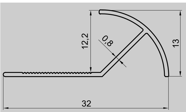
Teknik Çizim / Technical Drawing
