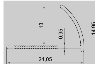
Teknik Çizim Technical Drawing
