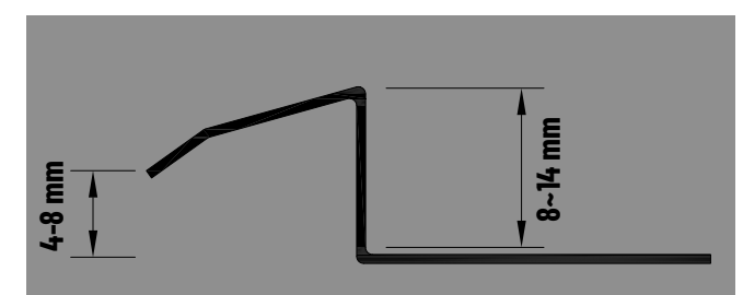
Teknik Çizim / Technical drawing
